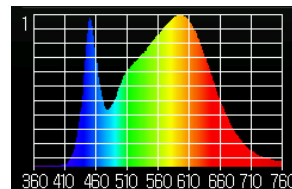
Спектр излучения
