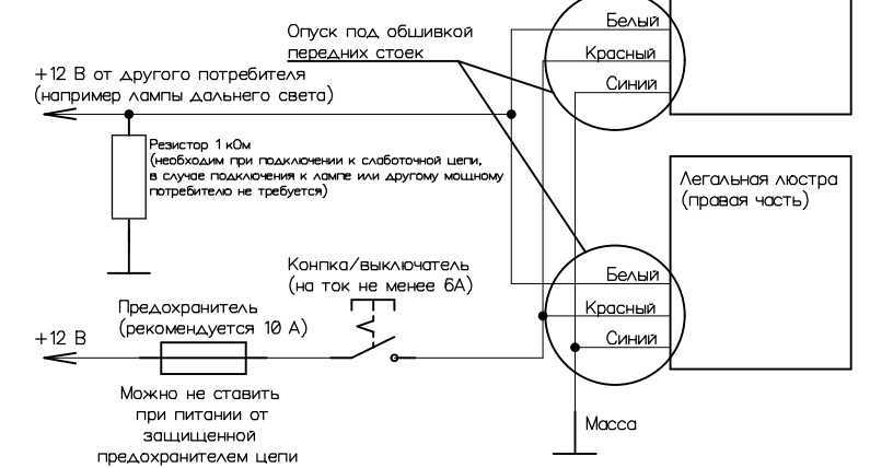
Схема подключения с использованием ШИМ-регулятора
