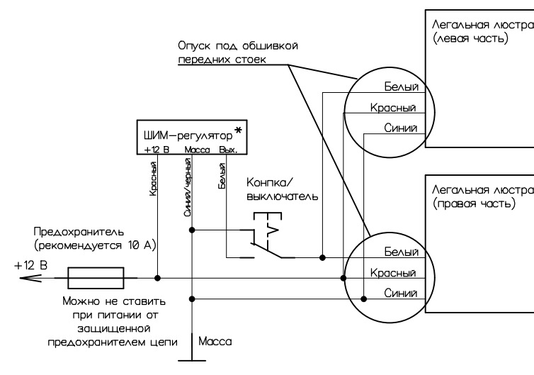
Схема подключения с управлением слаботочным переключателем и ШИМ-регулятором (в выключенном состоянии присутствует постоянное потребление тока не более 15 мА)
