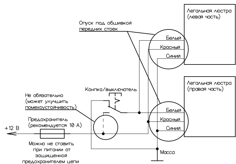
Схема подключения с управлением слаботочным переключателем (в выключенном состоянии присутствует постоянное потребление тока не более 10 мА)
