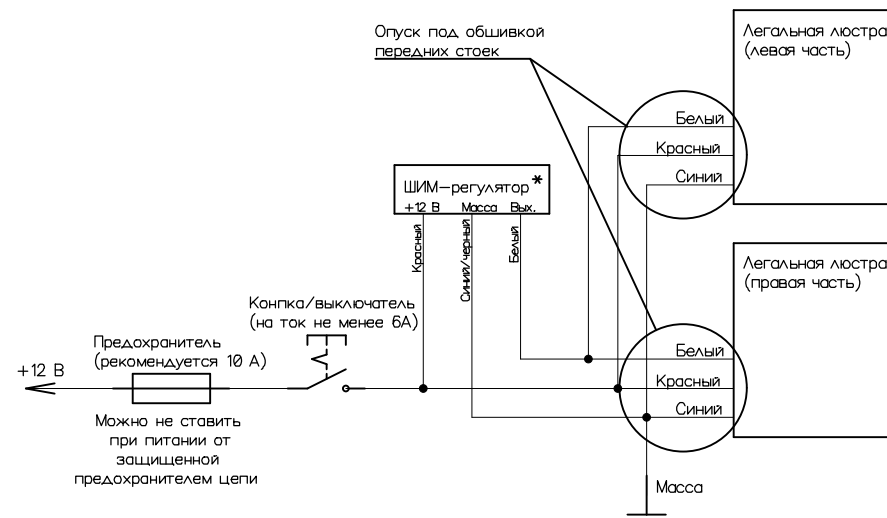
Схема подключения с использованием ШИМ-регулятора * цвета указаны дл регулятора нашего производства
