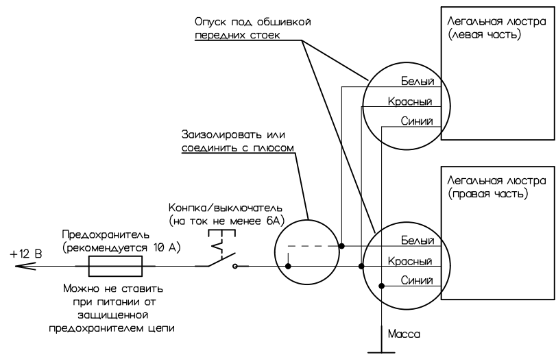
Схема подключения без использования регуляровки
